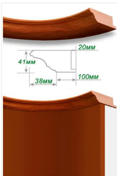
КАРНИЗ - ВОГНУТИЙ
