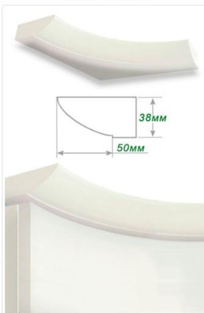
КАРНИЗ - ВОГНУТИЙ
