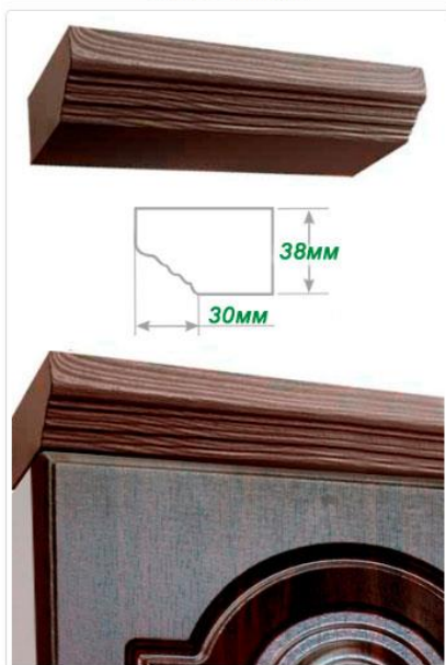
КАРНИЗ - ПРЯМИЙ
