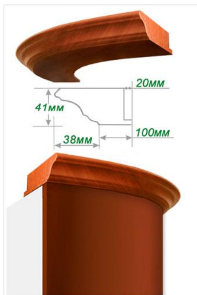
КАРНИЗ - ВИГНУТИЙ
