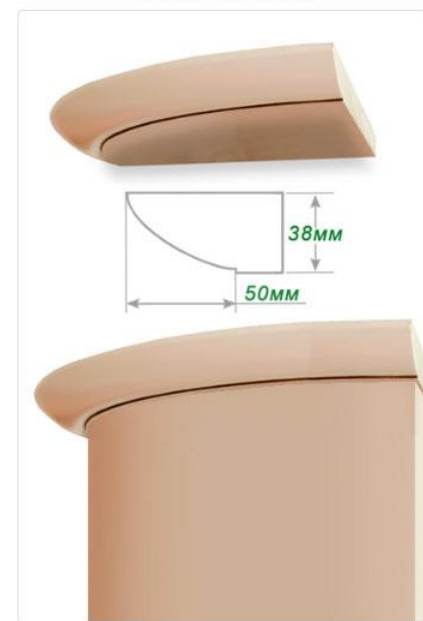
КАРНИЗ - ВИГНУТИЙ
