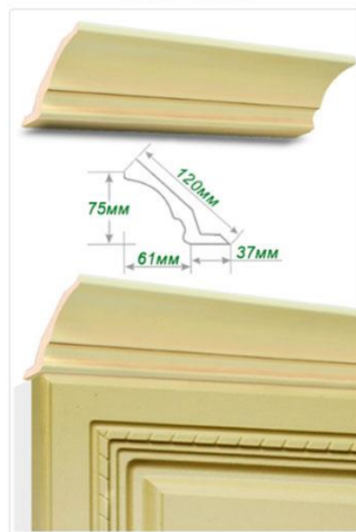
КАРНИЗ - ПРЯМИЙ
