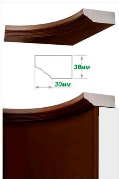
КАРНИЗ - ВОГНУТИЙ
